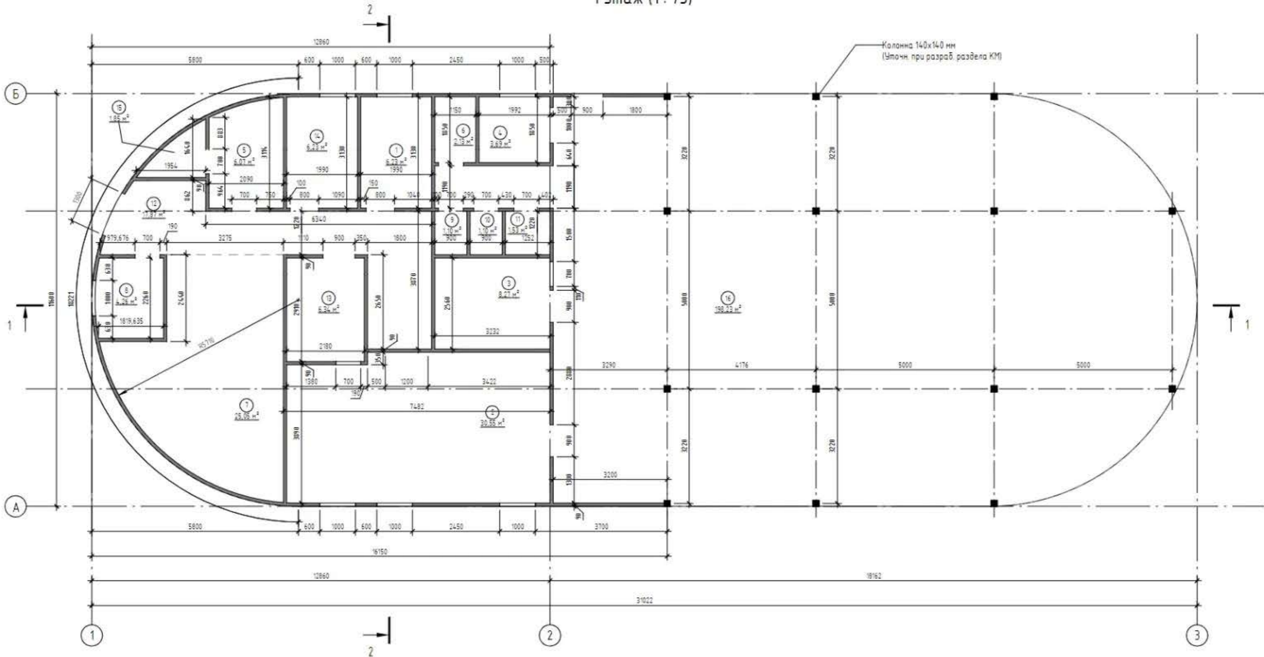
Экспликация помещений
