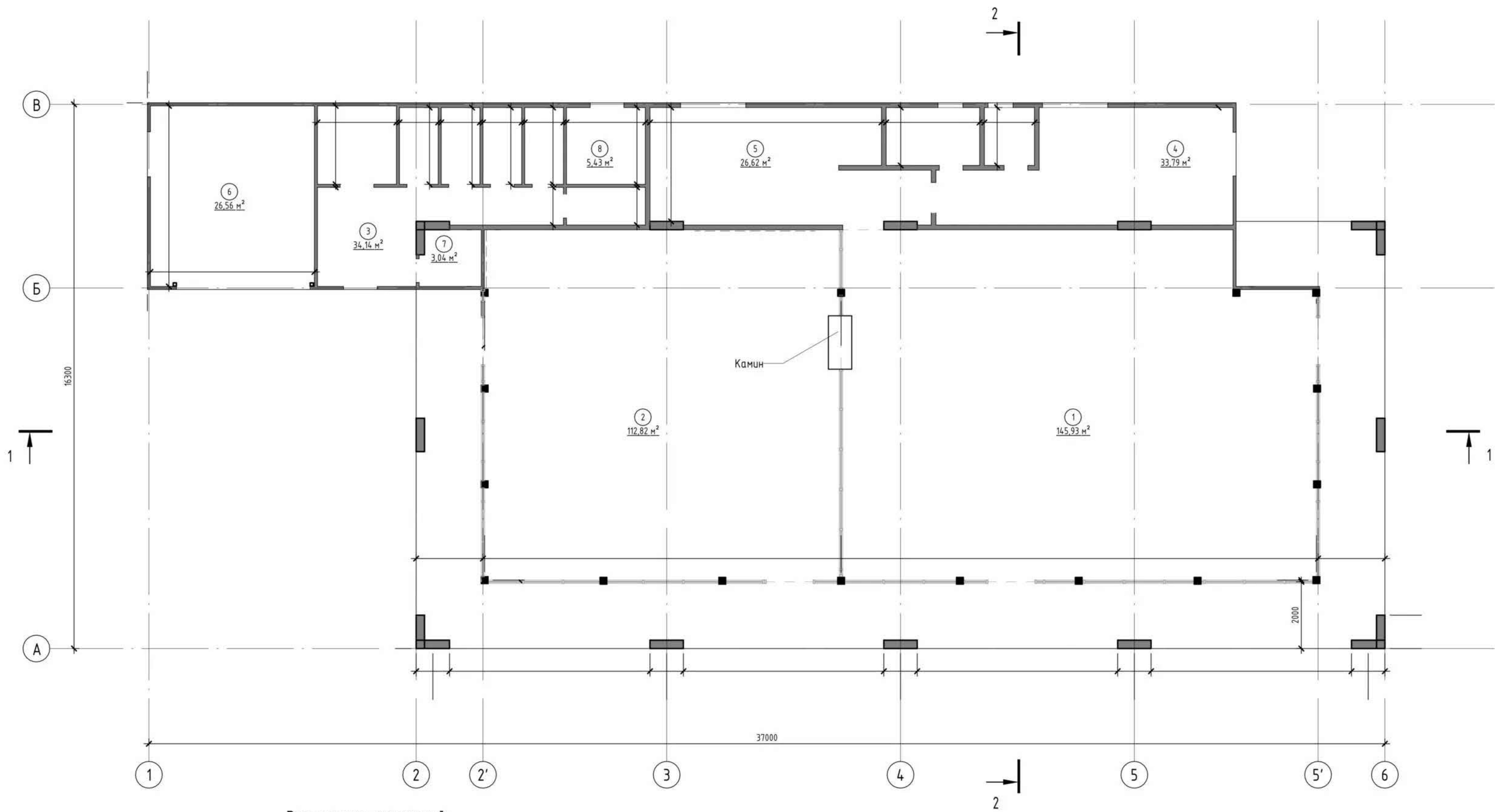
Экспликация помещений
