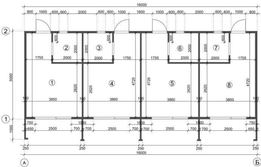
ПЛАН
