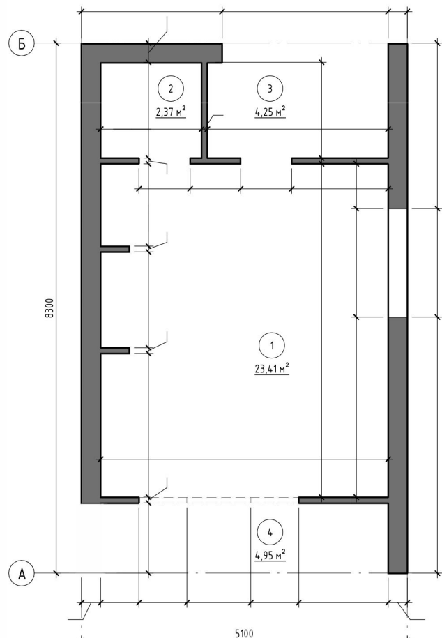
Экспликация помещений
