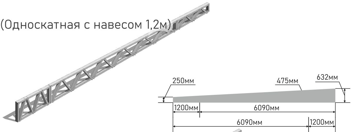
F06-8.49 (Односкатная 2 навеса по 1,2м)
