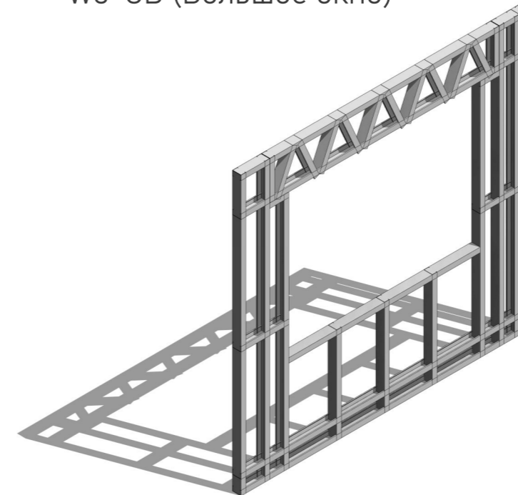
W3-OB (Большое окно)
