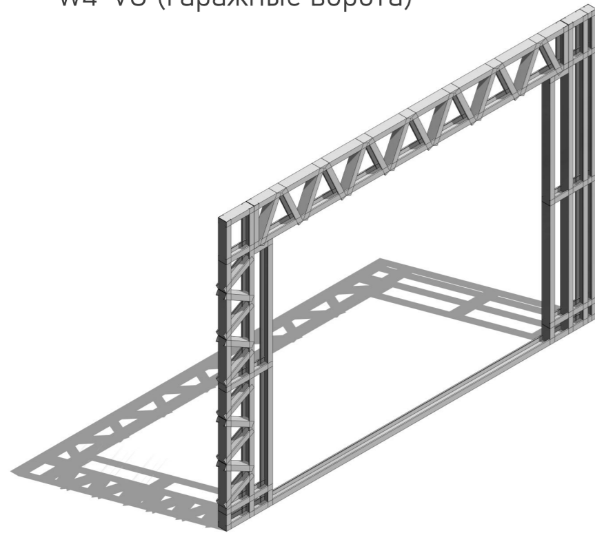
W4-VG (Гаражные ворота)
