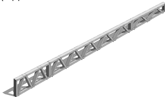
F03-5.49 (Односкатная 2 навеса по 1,2м)
