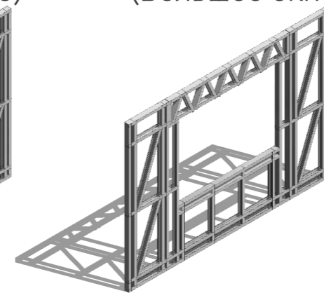
W4-OB (Большое окно)
