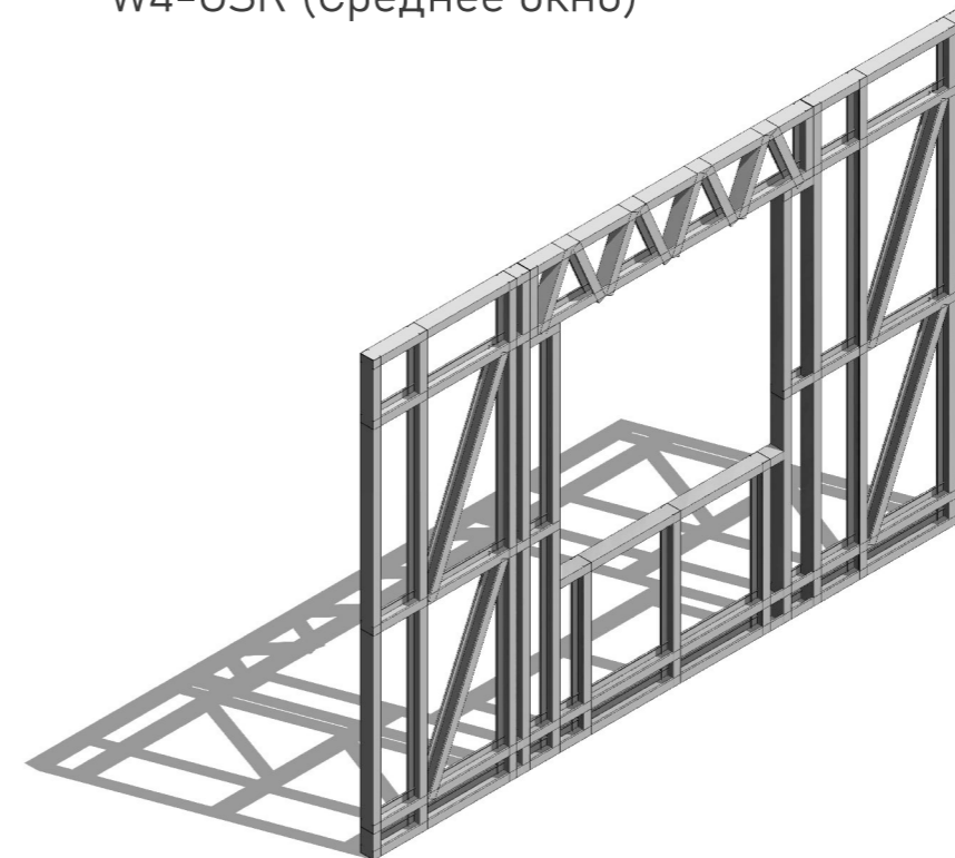
W4-OSR (Среднее окно)
