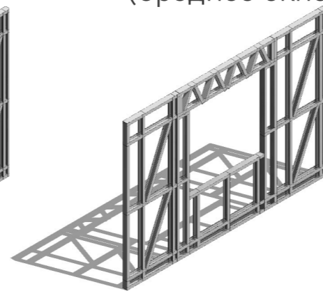
W4-OSR (Среднее окно)
