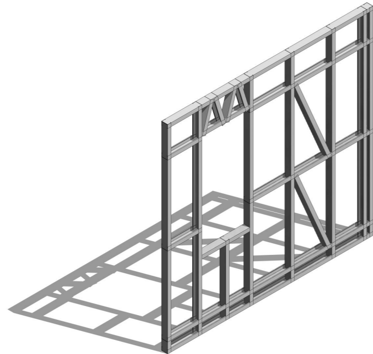
W3-OSR (Среднее окно)
