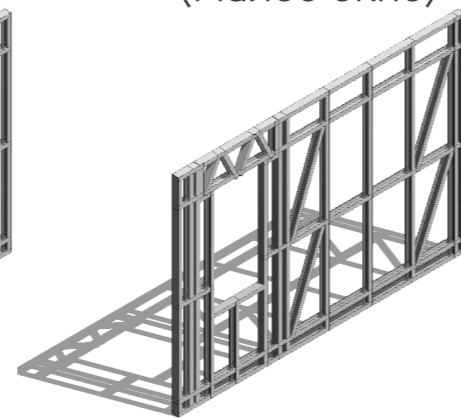
W4-OM (Малое окно)
