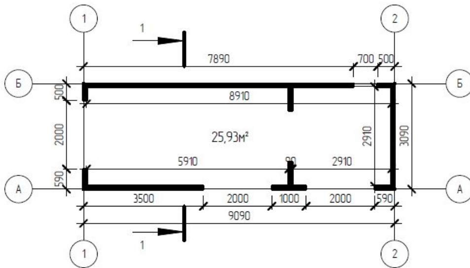
План 1 этажа
